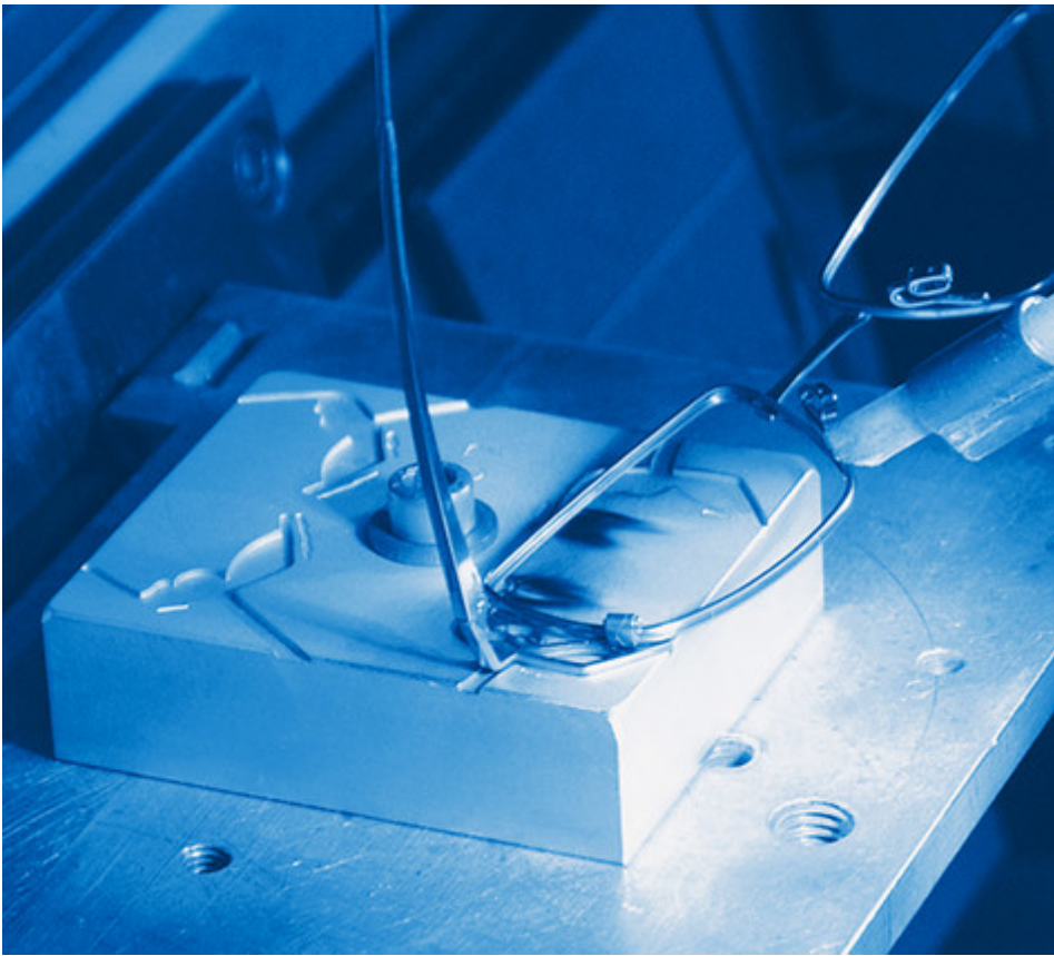
Brillenschweißverfahren
